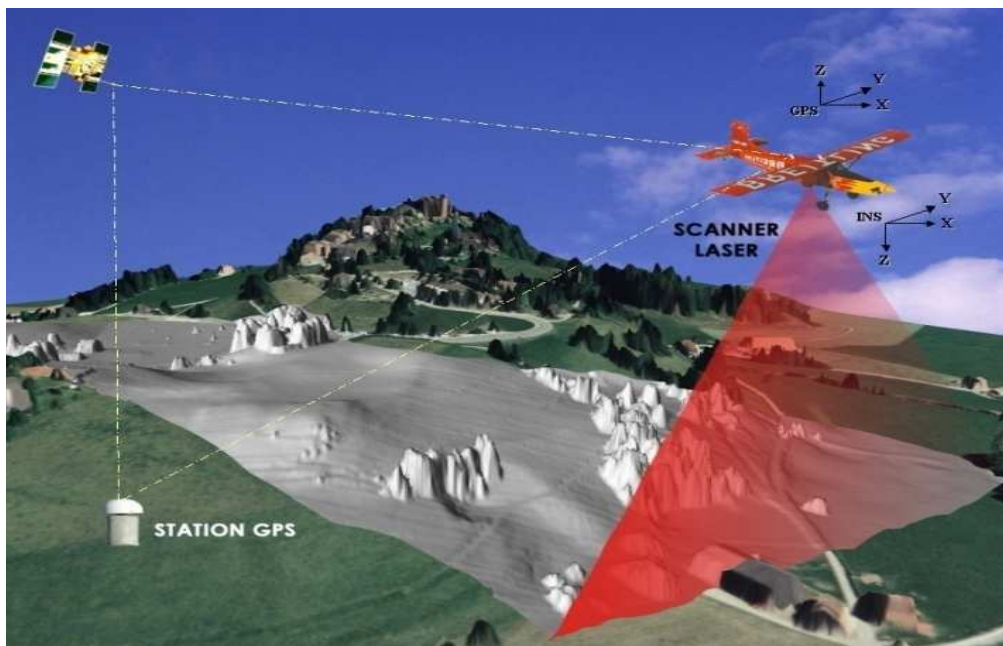
Figure 2 : Méthode d'acquisition par balayage laser (© SITN ( www.ne.ch/sitn ))
